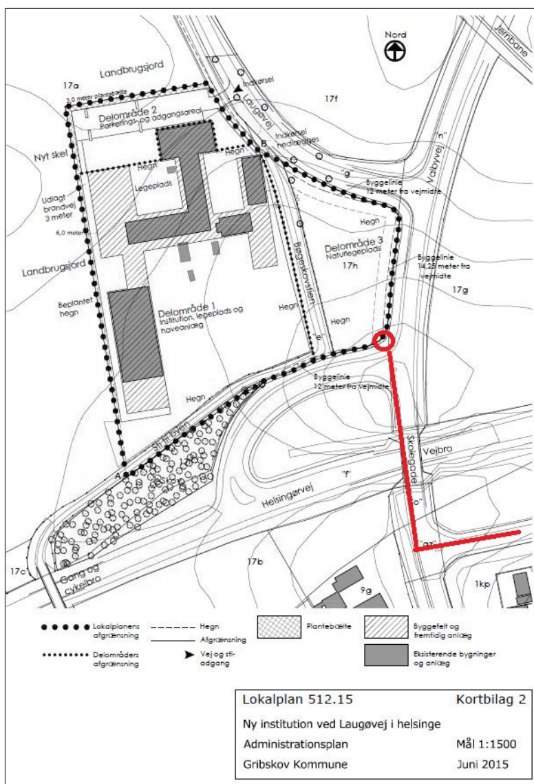
Figur 1. Oplandsgrænse vist med prikket signatur, afledning af spildevand vil følge rød linie
